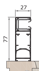
Führungsschienen RAFF S Schacht
