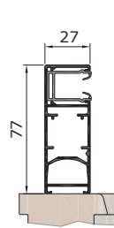
Führungsschienen RAFF S Putz
