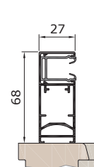
Führungsschienen RAFF S Schacht
