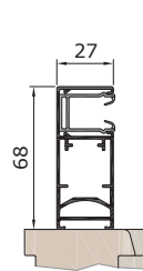
Führungsschienen RAFF S Blende
